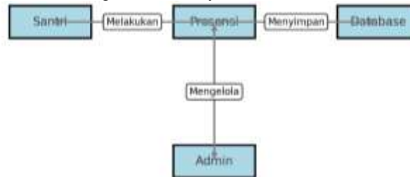
Gambar 4 ERD Proses Presensi Santri
