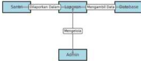
Gambar 6 ERD Proses Pembuatan Laporan
