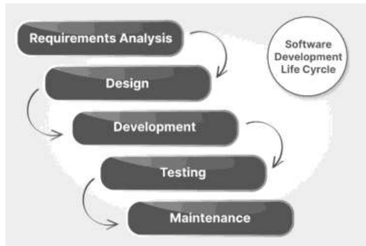
Gambar 1. Konsep Waterfall
